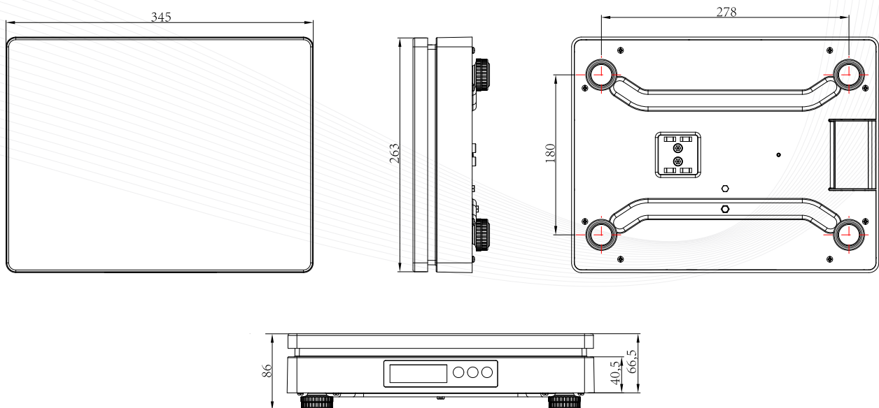
尺寸圖(mm)
